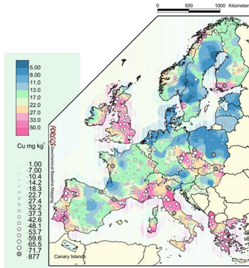
Figure 16. Distribution géographique du cuivre dans les sédiments des cours d'eau, d'après FOREGS.
