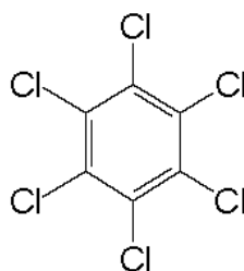
Formule de l'hexachlorobenzene
